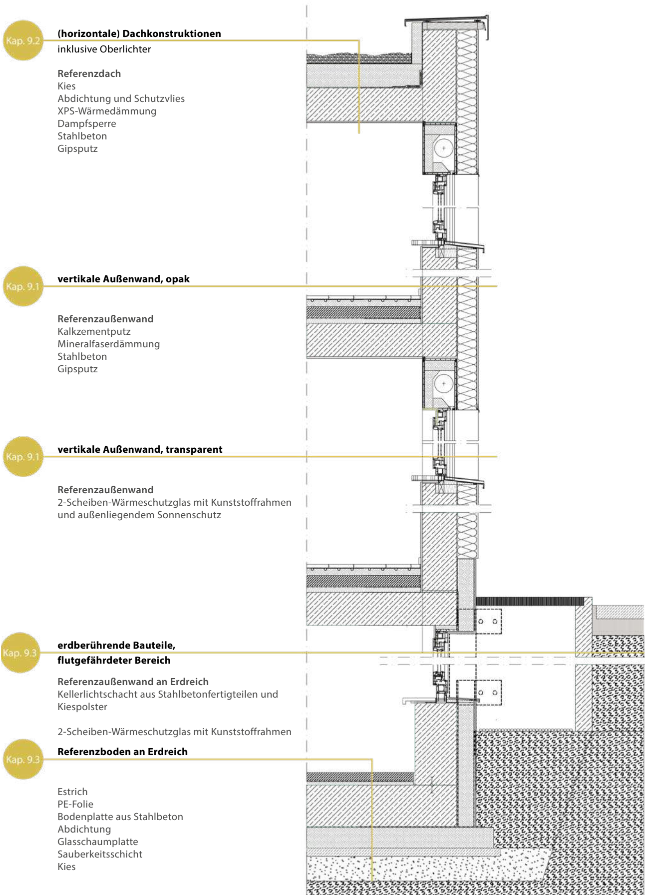
Abb. 17 Referenzbauteile sowie Verweise zu den Bauteilgruppen.
