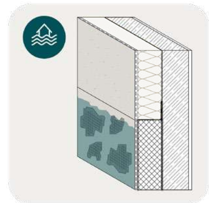
Abb. 80 Auswirkungen der Überflutung auf das Wärmedämmverbundsystem. Bauteilschäden infolge hoher hygrischer Belastung.
