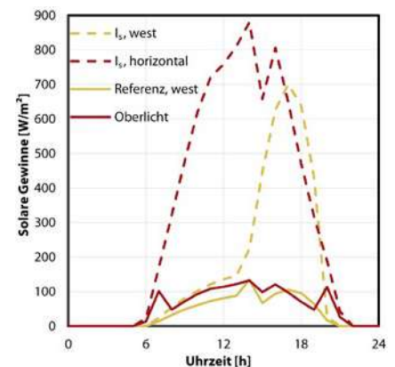
Abb. 78 Solarstrahlung ( I_s ) außen und solare Gewinne in Abhängigkeit der Zeit. Die Solarstrahlung außen west und die Solarstrahlung horizontal stellen die auf die vertikale bzw. horizontale Außenoberfläche auftreffende Sonneneinstrahlung dar. Die anderen Verläufe zeigen den solaren Energieeintrag in den Innenraum durch ein west- bzw. horizontal orientiertes Fenster.
