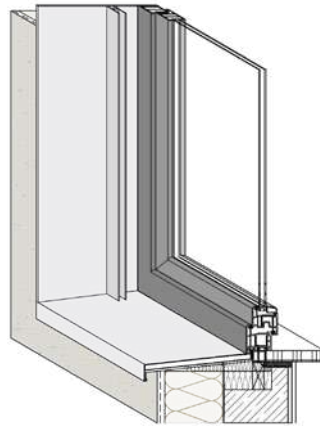
Abb. 58 Schnittansicht – Fenster.
