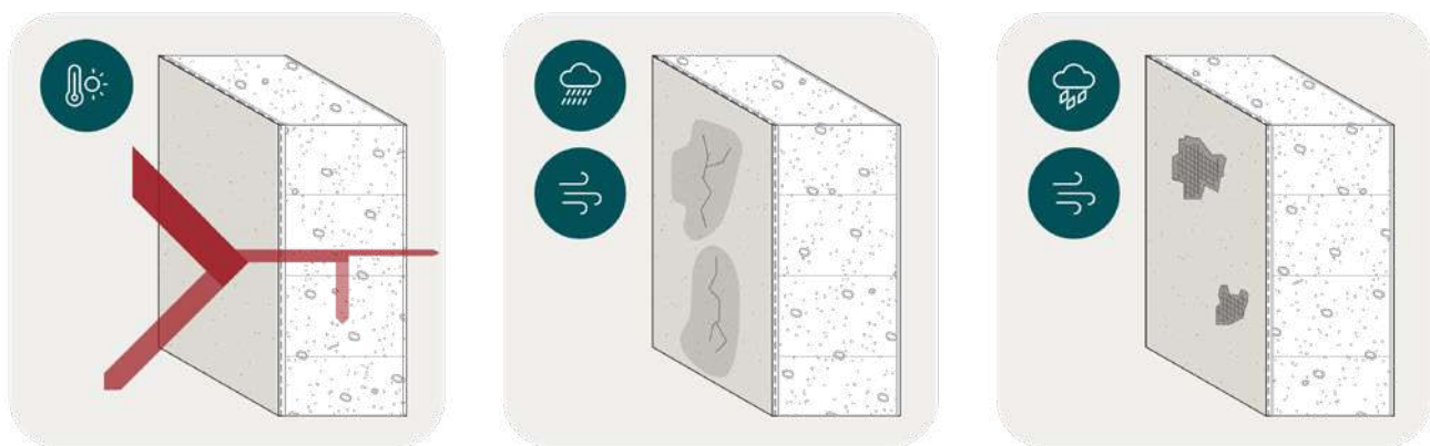
Abb. 51 Auswirkungen der Wetterelemente auf die Porenbetonkonstruktion. Links: Hitzeeintrag in das Bauteil. Mitte: Feuchteeintrag infolge Schlagregen. Rechts: Schäden am Putzsystem infolge Hagel und Sturm.
