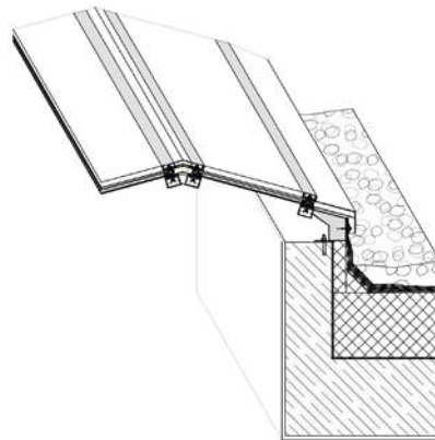
Abb. 76 Schnittansicht – Dachoberlicht.
