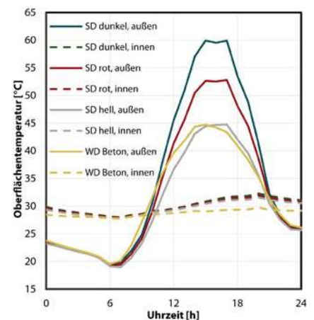
Abb. 75 Oberflächentemperaturverläufe außenseitig sowie innenseitig der Referenz- und Satteldachflächen in Abhängigkeit der Ziegelfarbe.
