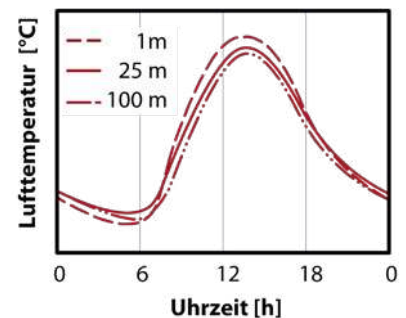
Abb. 8 Darstellung des schematischen Temperaturverlaufs an einem strahlungsreichen, wolkenlosen Tag in verschiedenen Höhen über dem Boden (Oke, T. R. 1997).
