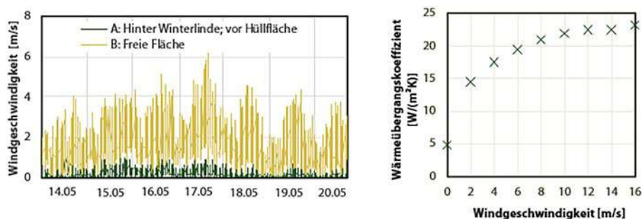
Abb. 36 Links: Vergleich der Windgeschwindigkeit zwischen Winterlinde und Fassadenoberfläche (Graph A) sowie einer freien Fläche (Graph B) bei einer Messreihe im Mai 2020 in Stuttgart-Vaihingen. Rechts: Einfluss der Windgeschwindigkeit auf den konvektiven Wärmeübergangskoeffizienten nach (Mayer, E. et al. 2018).
