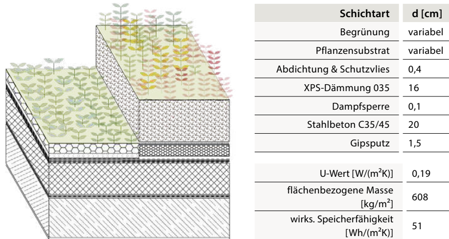
Abb. 70 Schnittansicht – Gründach extensiv und intensiv.
