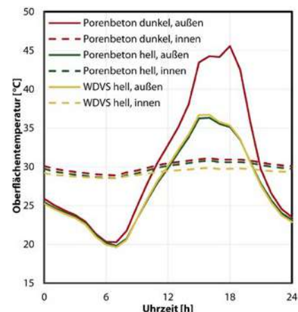
Abb. 52 Oberflächentemperaturverläufe außenseitig sowie innenseitig über einen Tag in Abhängigkeit der Putzfarbe.
