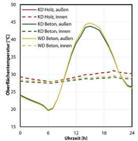
Abb. 69 Oberflächentemperaturverläufe außenseitig sowie innenseitig der Referenz- und Kaltdachflächen.
